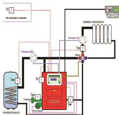
Katilo pajungimo schema
