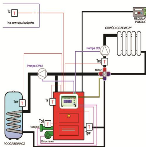
Katilo pajungimo schema
