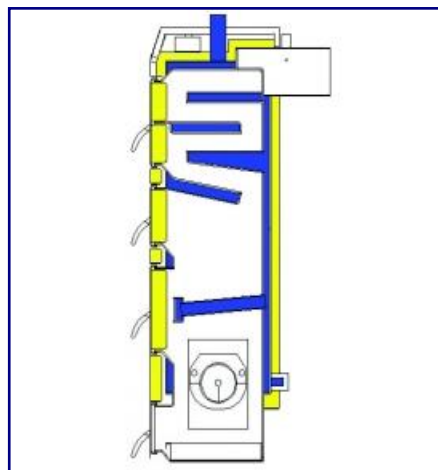
SD DUO šilumokaitis
